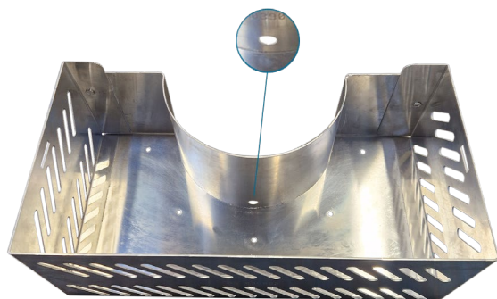
Limiteur de débit / déversoir avec orifice(s) d'évacuation calibré(s) et surverse
